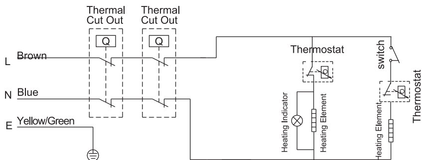
СХЕМА ЕЛЕКТРОПРОВОДКИ
